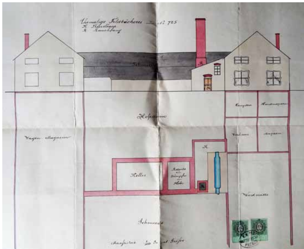
📍 Plán instalace parního stroje v domě čp. 725, 1882. SOKA Přerov
